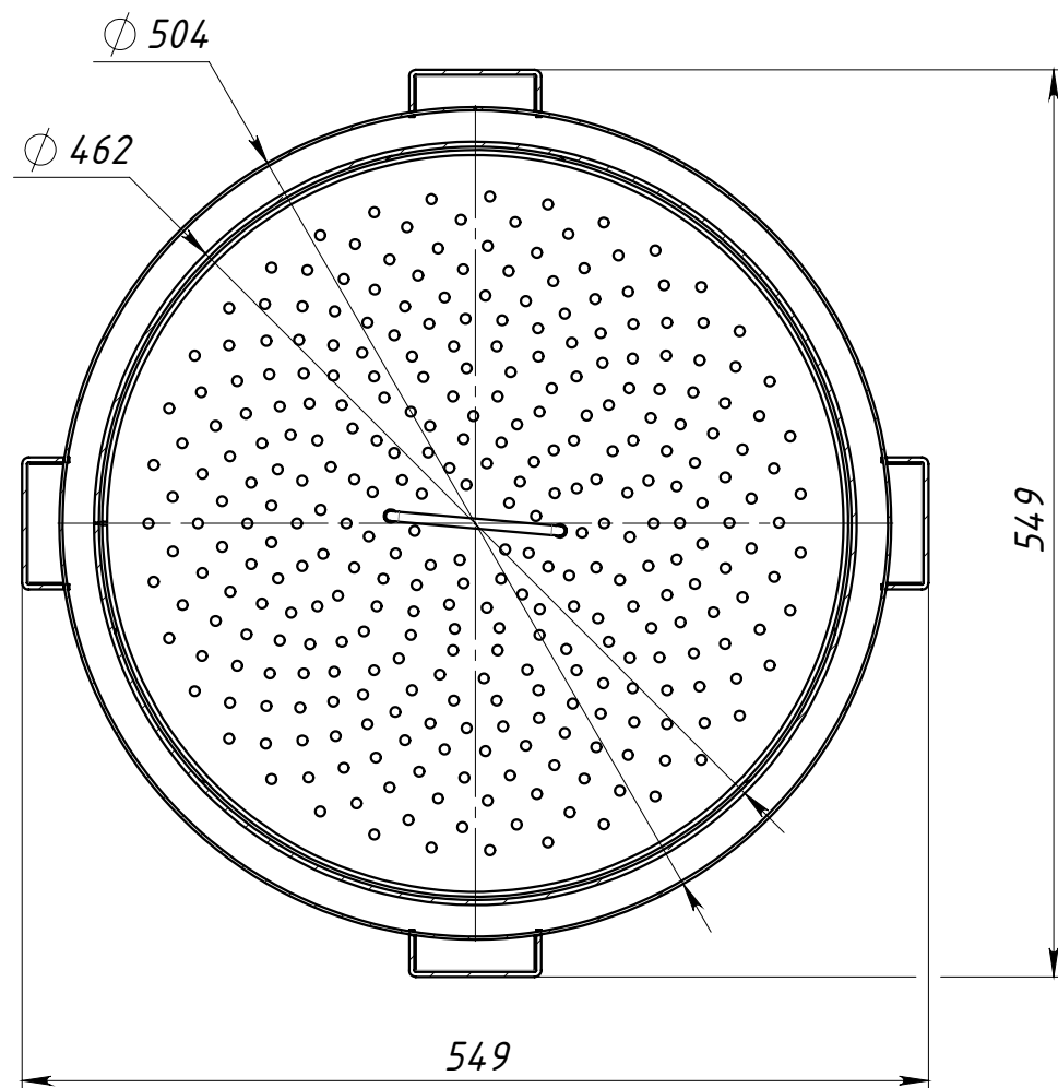
Б-Б (1 : 5)
